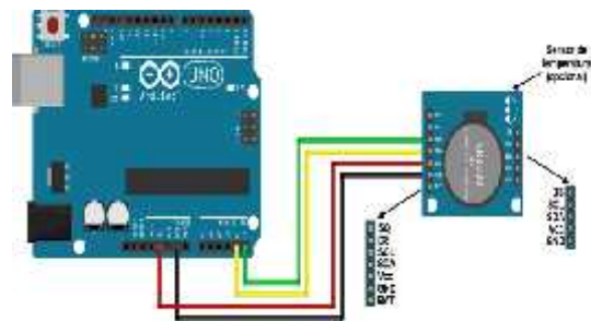
Gambar 9. RTC DS1307
