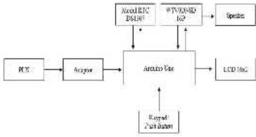
Gambar 6. Desain Sistem Bel Sekolah Otomatis
