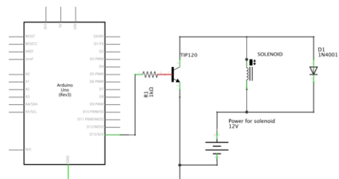
Gambar 4 Skema Pengujian Arduino dengan Driver Solenoid Door Lock
