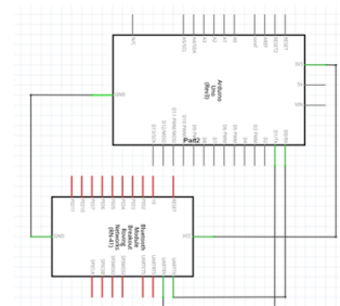
Gambar 7 Skema Pengujian Arduino dengan Modul HC-05
