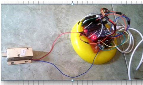
Gambar 5 Hasil Pengujian Arduino dengan Solenoid Door Lock
