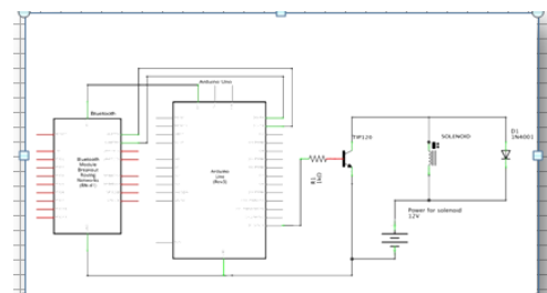
Gambar 9 Skema Pengujian Arduino dengan Modul HC-05 dan Solenoid Door Lock
